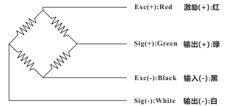
Wiring Diagram/接线图
