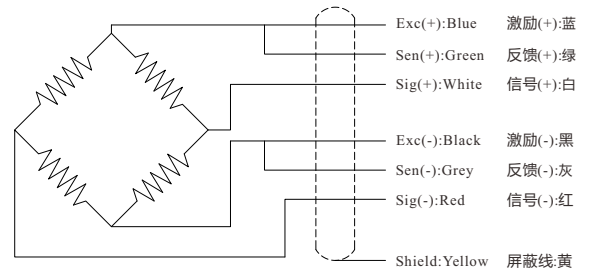
Wiring Diagram/接线图
